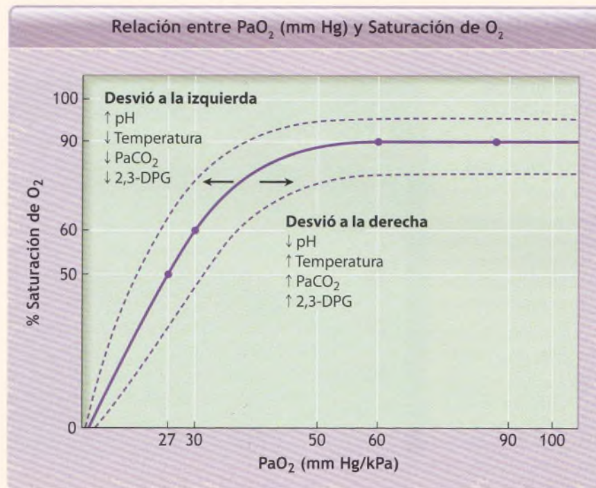
■ FIGURA II-2 Relación entre presión parcial de oxígeno en sangre arterial ( \text{PaO}_2 ) y % Saturación de \text{O}_2 .
